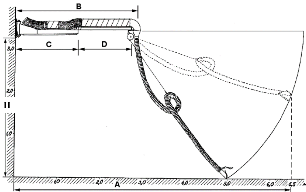
Вытяжное устройство
